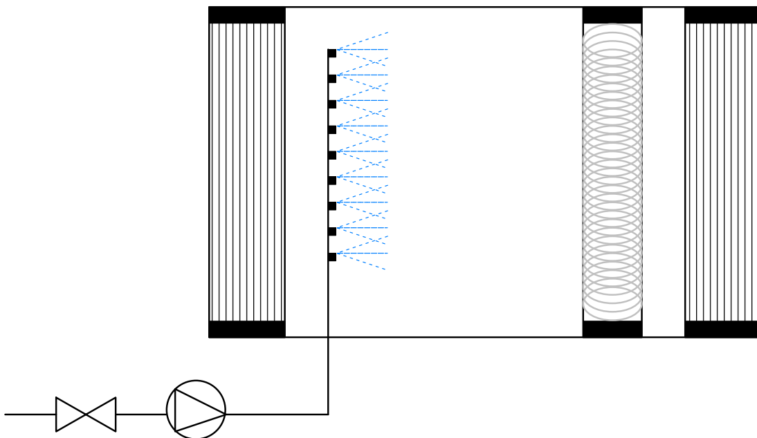
Abbildung 2: Fließbild Jetvap
